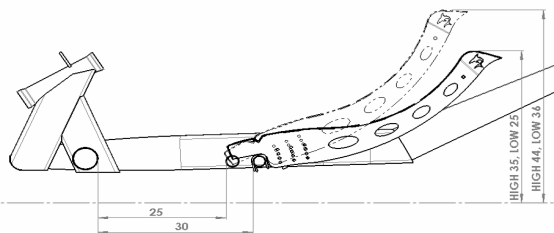
Positie diepte rugleuning 250 mm (SRK030003) of 300 mm (SRK030004)
